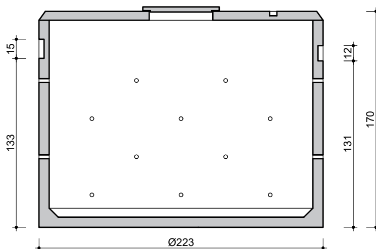
DOORSNEDE COUPE
