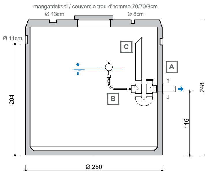
DOORSNEDE COUPE
