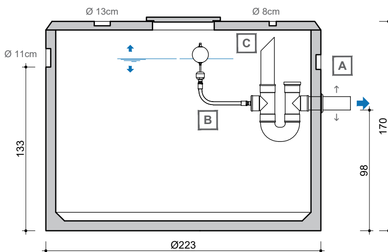
DOORSNEDE COUPE
