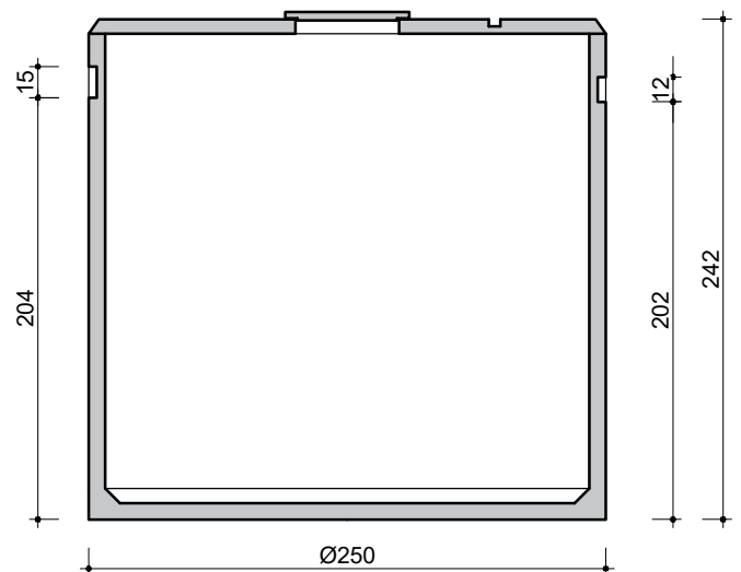
DOORSNEDE COUPE
