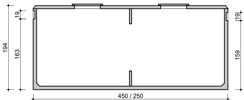
DOORSNEDE COUPE
