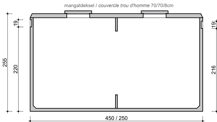
DOORSNEDE COUPE
