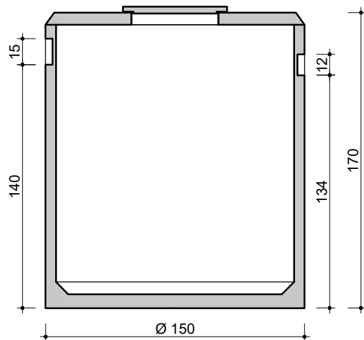
DOORSNEDE COUPE
