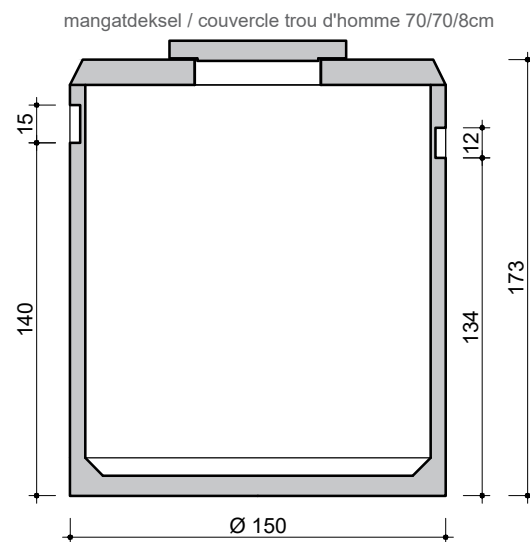
DOORSNEDE COUPE
