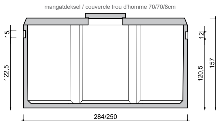
DOORSNEDE COUPE
