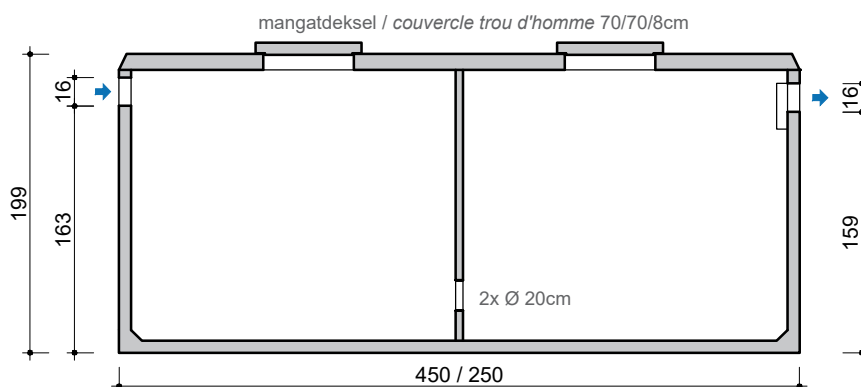
DOORSNEDE COUPE
