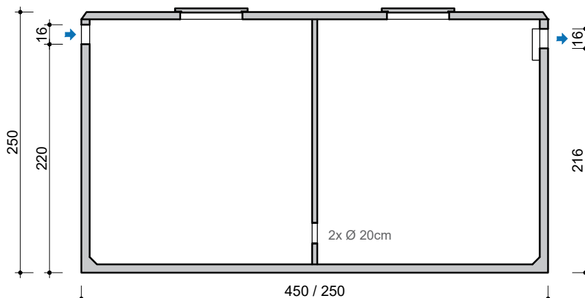
DOORSNEDE COUPE
