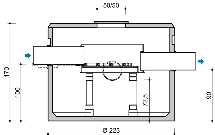
DOORSNEDE COUPE
