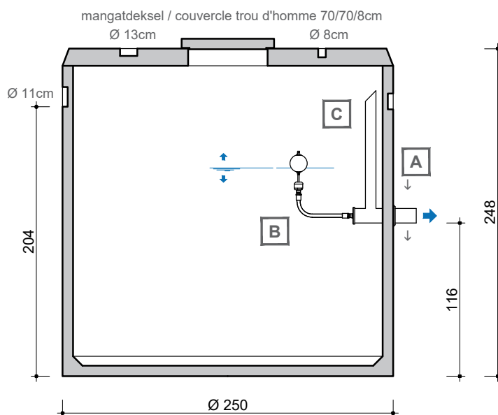
DOORSNEDE COUPE
