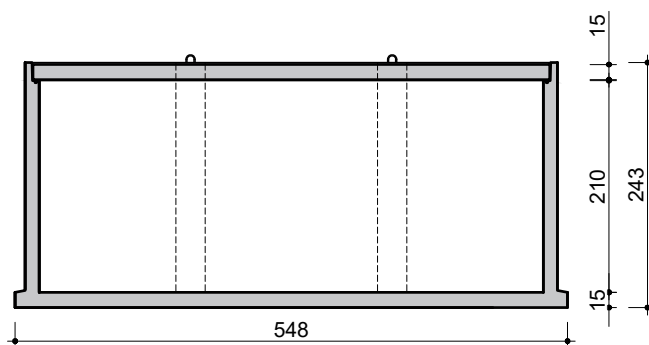
LANGSE DOORSNEDE COUPE LONGITUDINALE
