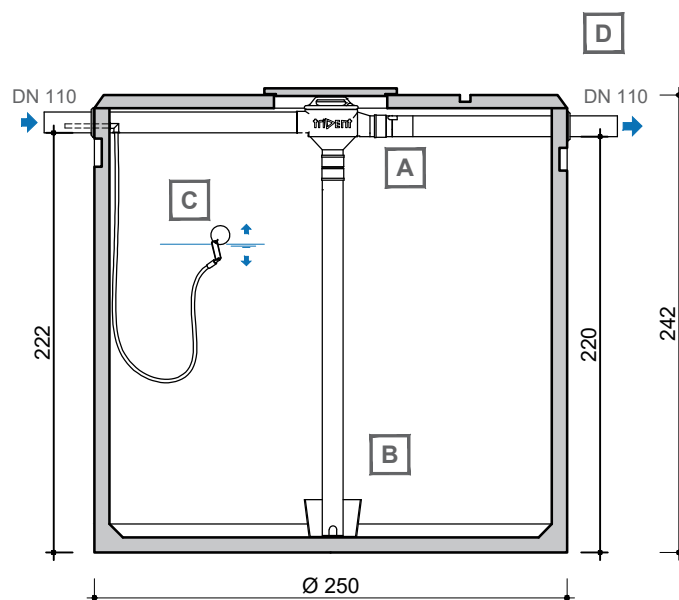
DOORSNEDE COUPE
