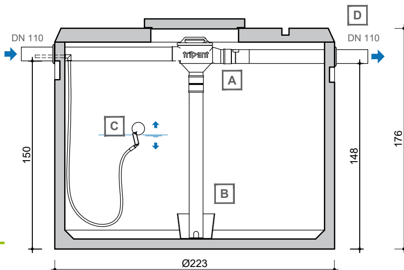
DOORSNEDE COUPE
