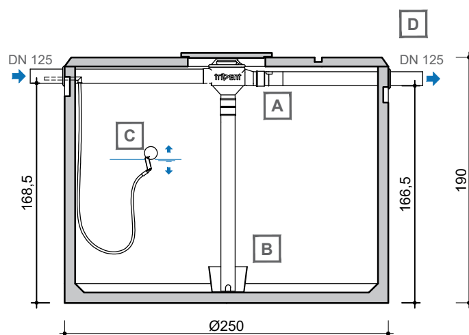
DOORSNEDE COUPE
