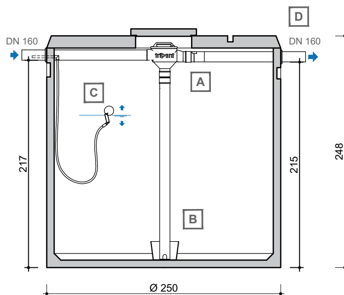
DOORSNEDE COUPE
