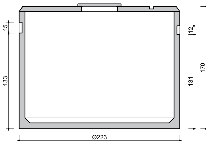
DOORSNEDE COUPE
