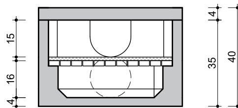
DOORSNEDES COUPES
