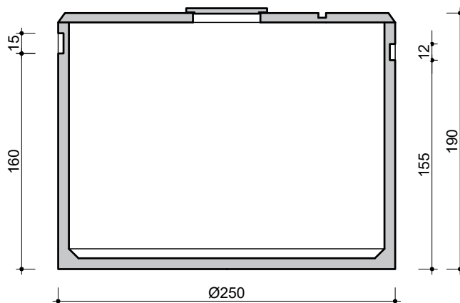
DOORSNEDE COUPE
