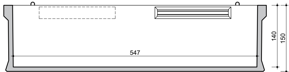
LANGSE DOORSNEDE COUPE LONGITUDINALE
