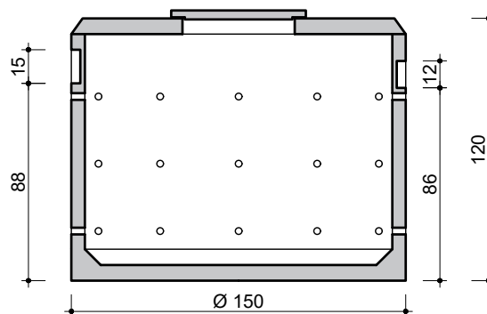
DOORSNEDE COUPE
