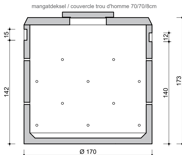
DOORSNEDE COUPE
