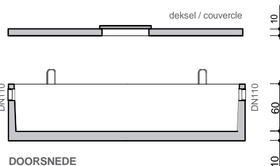
DOORSNEDE COUPE
