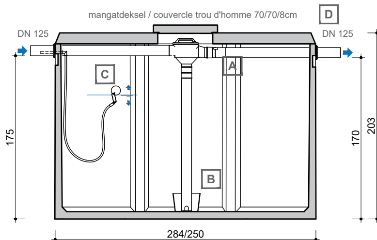
DOORSNEDE COUPE
