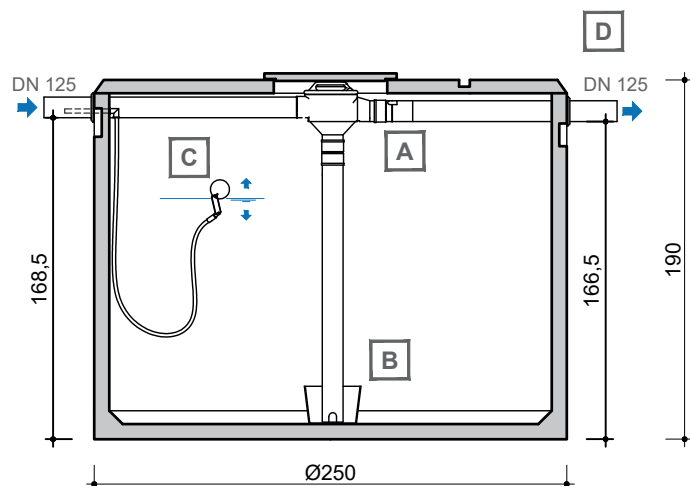
DOORSNEDE COUPE
