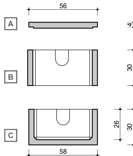
DOORSNEDES COUPES
