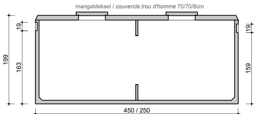
DOORSNEDE COUPE
