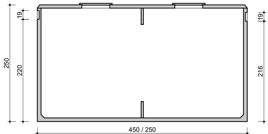
DOORSNEDE COUPE
