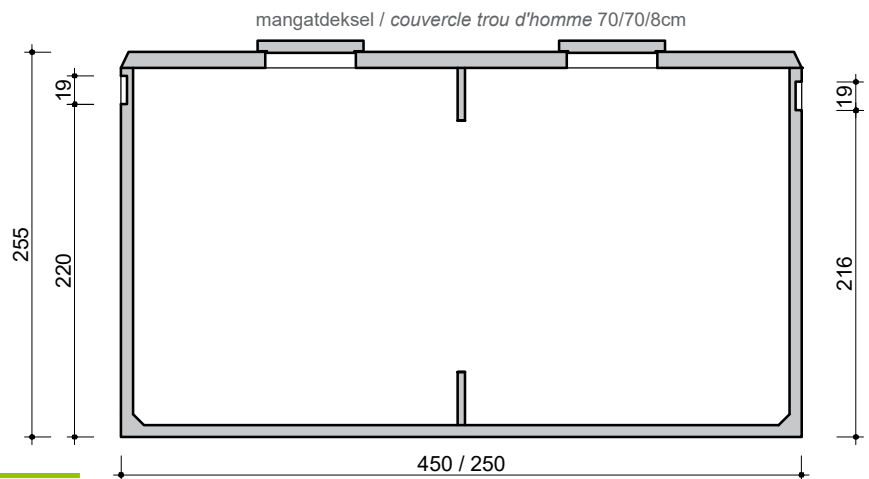
DOORSNEDE COUPE
