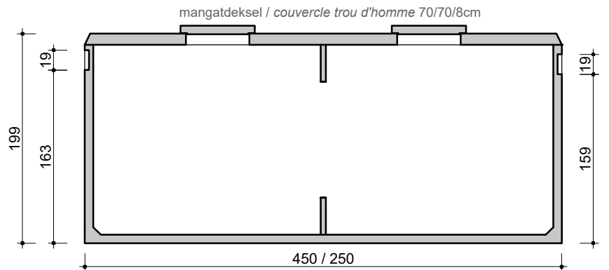
DOORSNEDE COUPE
