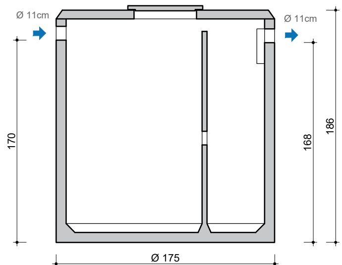
DOORSNEDE COUPE
