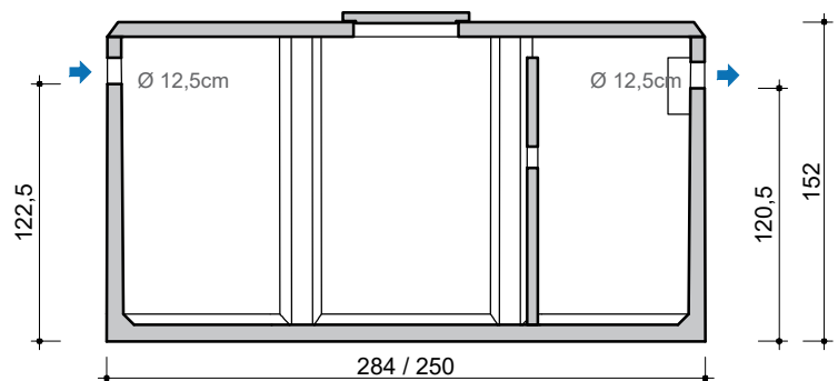
DOORSNEDE COUPE
