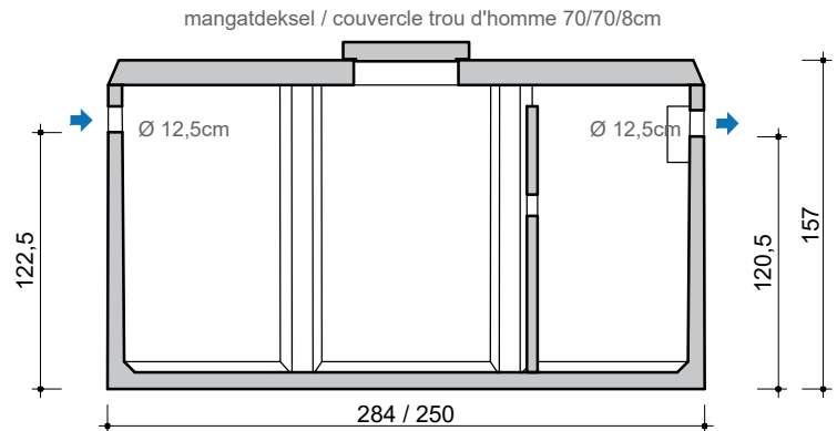
DOORSNEDE COUPE
