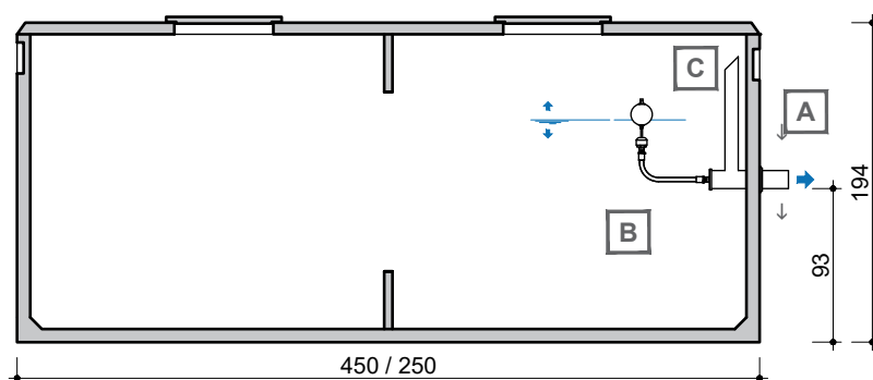
DOORSNEDE COUPE
