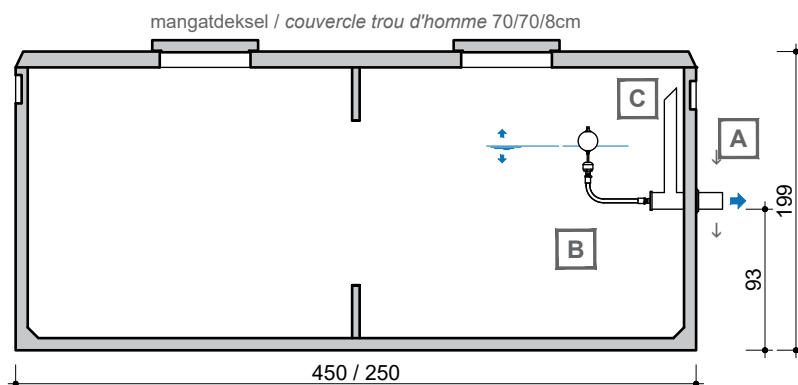
DOORSNEDE COUPE
