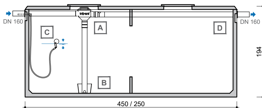
DOORSNEDE COUPE
