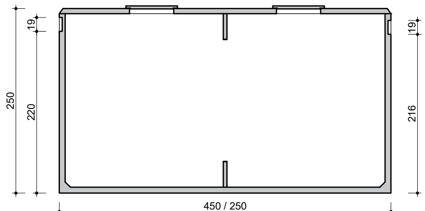
DOORSNEDE COUPE
