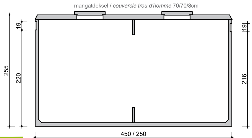
DOORSNEDE COUPE
