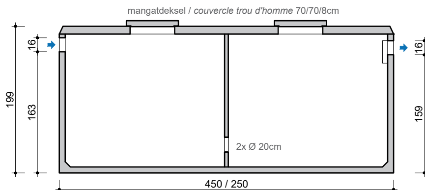
DOORSNEDE COUPE
