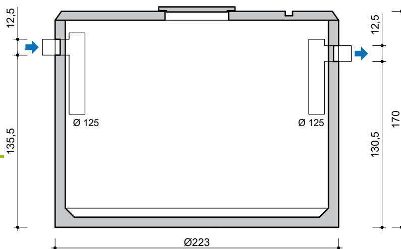
DOORSNEDE COUPE
